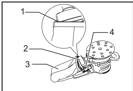
► 1. Crochet 2. Raccord à poussières 3. Sac à poussières 4. Bouton-poussoir
