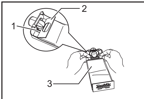
► 1. Ranura 2. Cartón de fijación frontal 3. Cara frontal de bolsa recolectora de polvo
