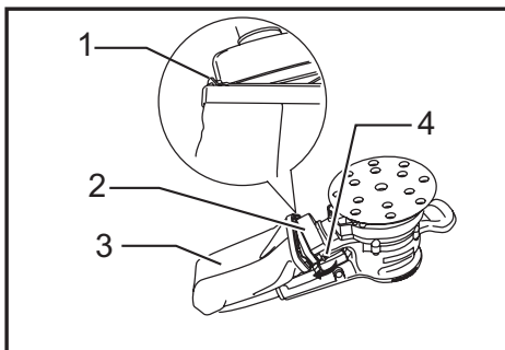
► 1. Hook 2. Dust nozzle 3. Dust bag 4. Push button
