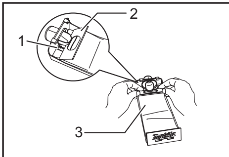
► 1. Rainure 2. Carton de fixation avant 3. Face avant du sac à poussières en papier
