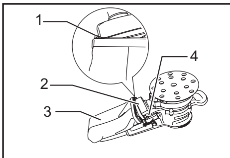
► 1. Gancho 2. Boquilla para polvo 3. Bolsa para polvo 4. Botón pulsador
