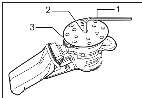
► 1. Llave hexagonal 2. Tornillo 3. Almohadilla
