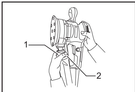
► 1. Raccord à poussières 2. Bouton-poussoir
